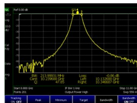
Использование маркеров для измерения полосы пропускания и добротности упрощает процесс тестирования и настройки фильтра
